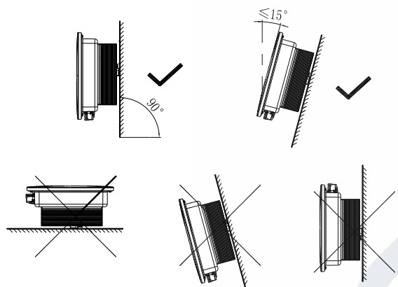
Obr. 5.1 Schéma instalace
