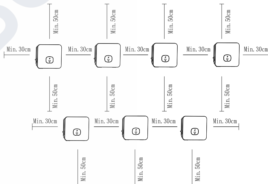
Obr. 5.2 Instalační rozměry pro více střídačů
