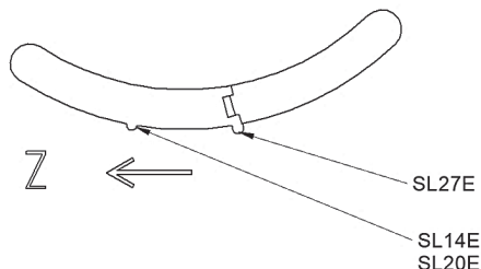
Obr. 11 Nastavení terciálního vzduchu u kotle SL14E, SL20E a SL27E.
