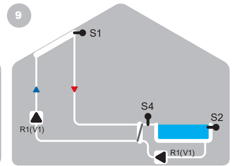
Solární systém s bazénem a výměníkem
