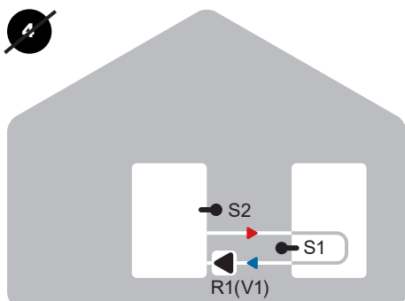
Předávání tepla mezi zásobníky
