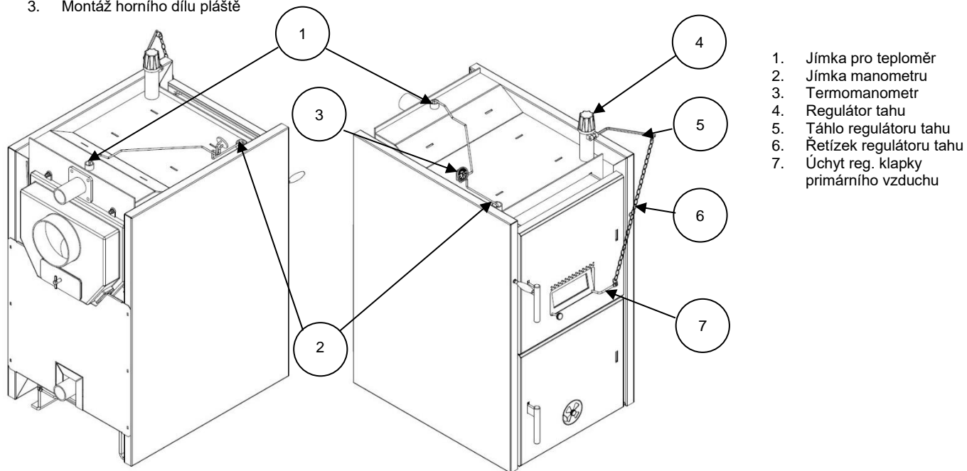
Obr.17 Instalace termomanometru a regulátoru tahu
